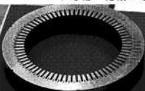
ハイブリッド車用モーターコア、外径30mm以下の高精度部品
